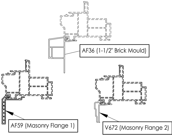
OPTIONAL COSMETIC FLANGES
